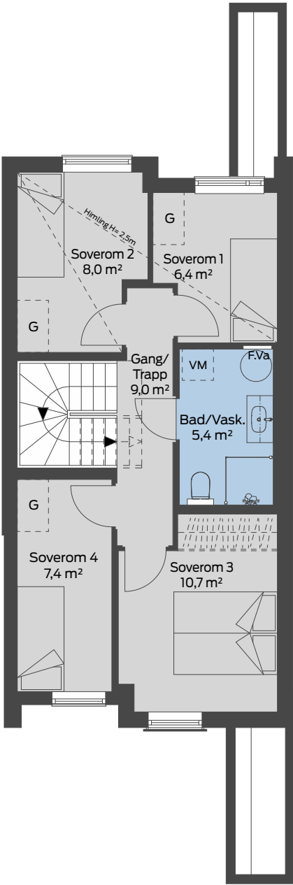
2. etasje
