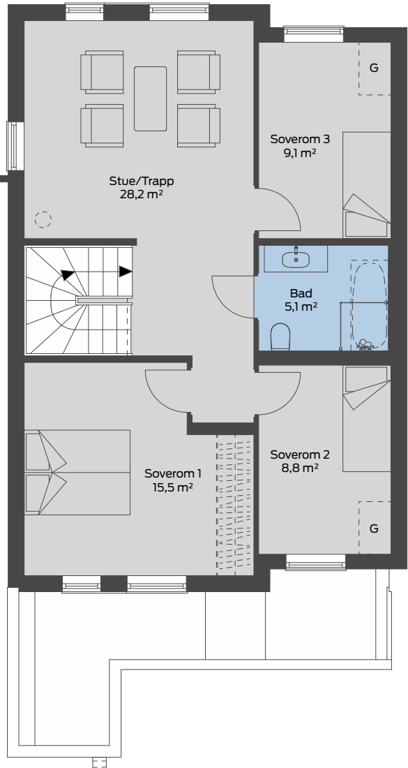
2. Etasje
