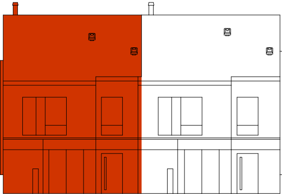
Fasade Sør-Øst
