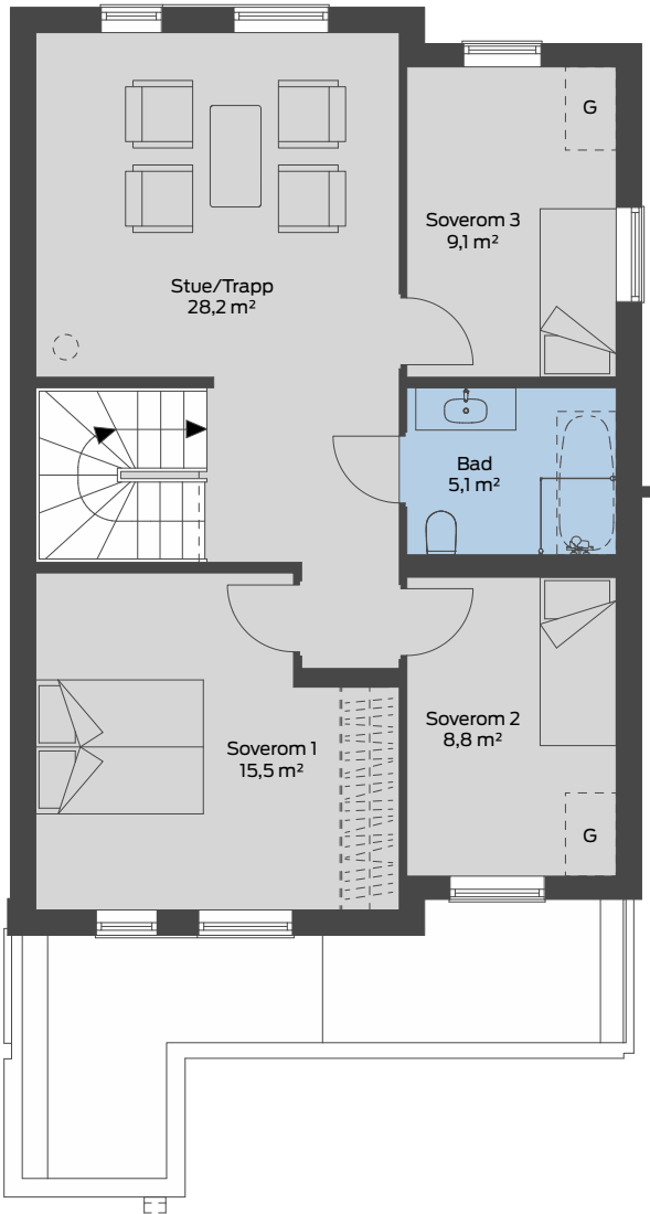
2. Etasje
